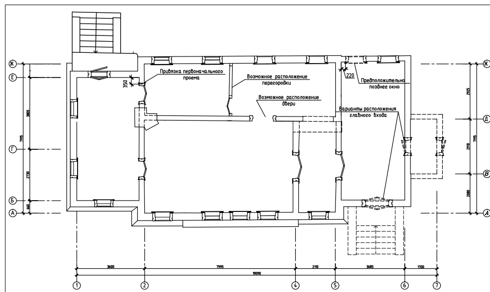
Предполагаемая планировка дома на первом этапе строительства.
