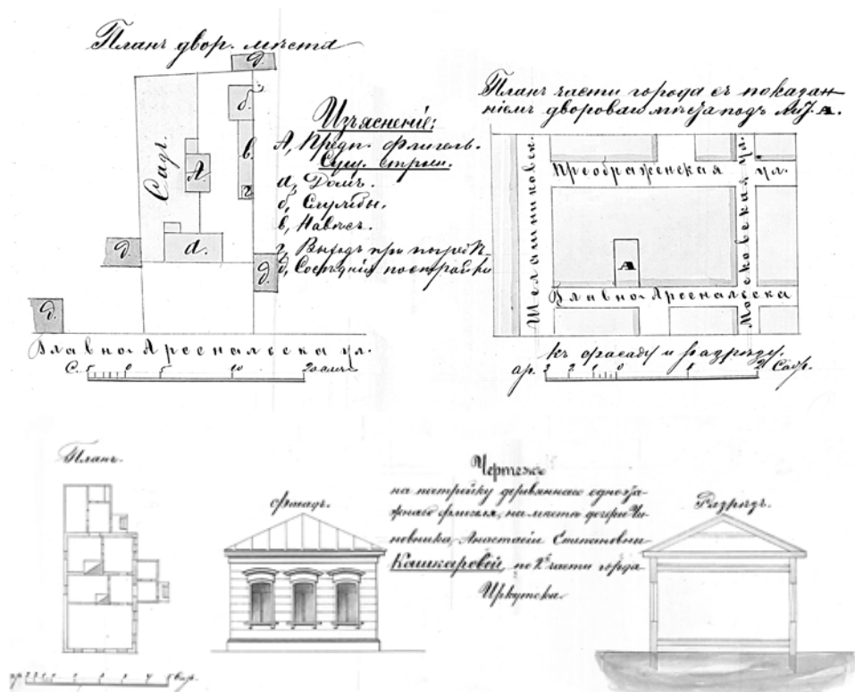
План дворового места и положение в квартале усадьбы А.С. Кашкаровой (вверху). Чертеж на постройку деревянного одноэтажного флигеля в усадьбе А.С. Кашкаровой (внизу). 1880. ГАИО
