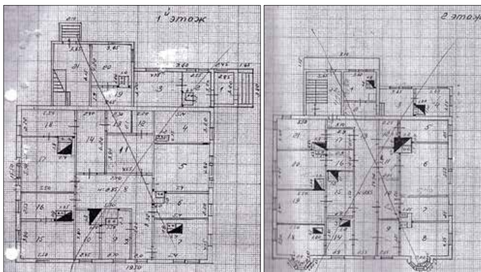
План первого и второго этажей дома Волконских. 1958
